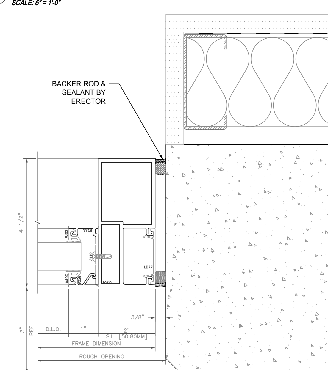
6 TRANSOM @ JAMB DETAIL SCALE: 6" = 1'-0"
