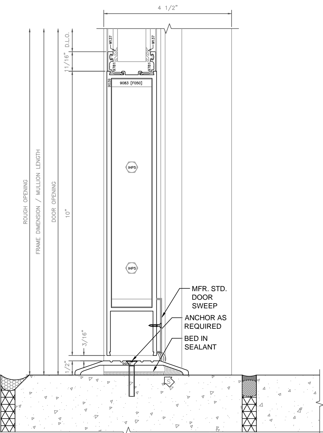
2 THRESHOLD DETAIL SCALE: 6" = 1'-0"
