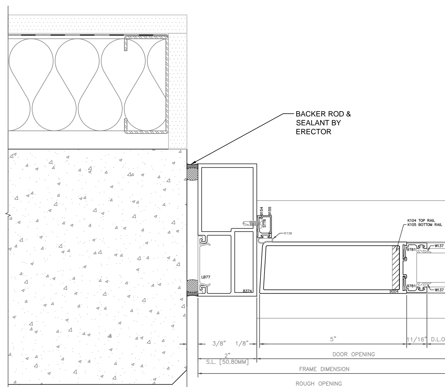
7 DOOR JAMB DETAIL SCALE: 6" = 1'-0"
