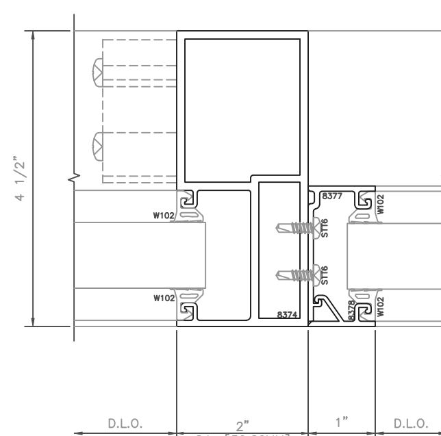
5 TRANSOM DETAIL SCALE: 6" = 1'-0"
